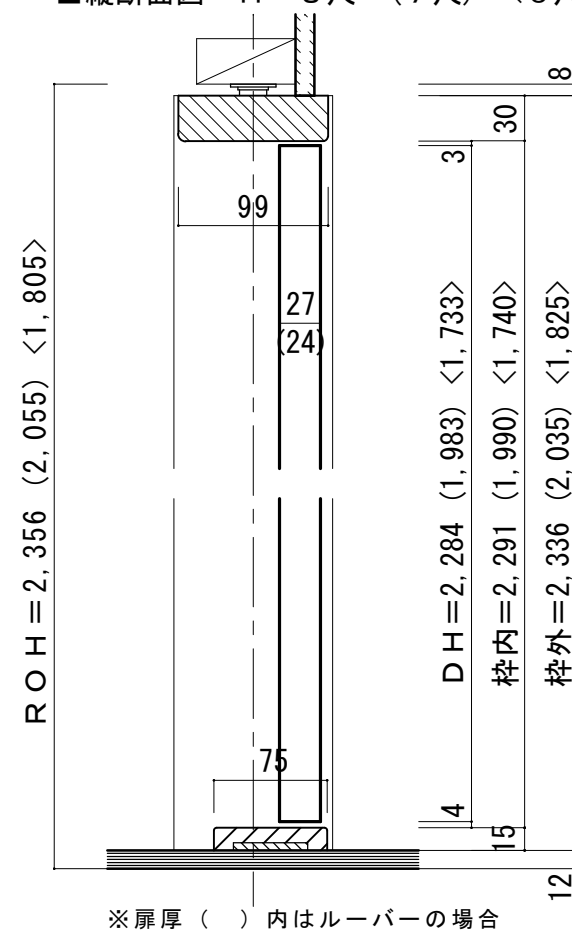
■縦断面図 H=8尺 (7尺) <6尺>
