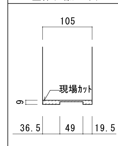
豎杵下端加工圖
