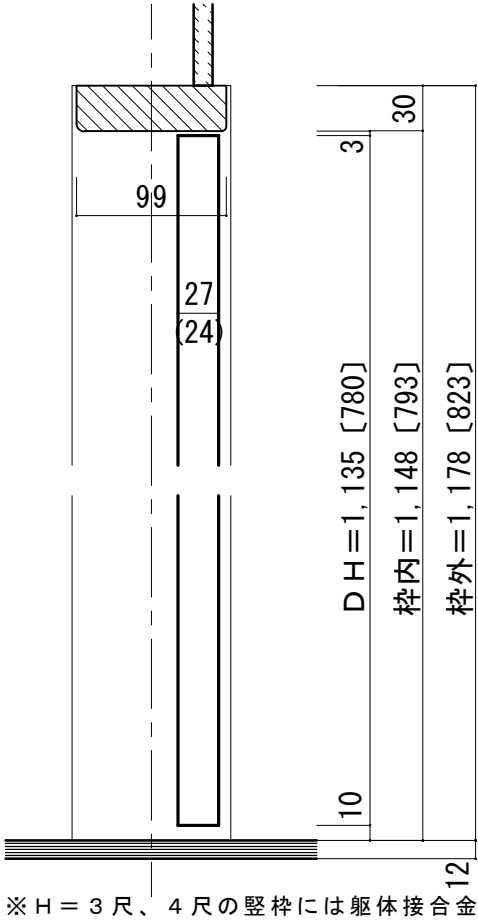
■縦断面図 H=4尺 [3尺]
