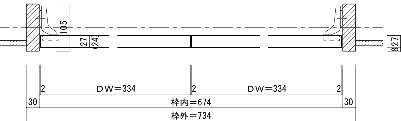
■横断面図 H=4尺、3尺
