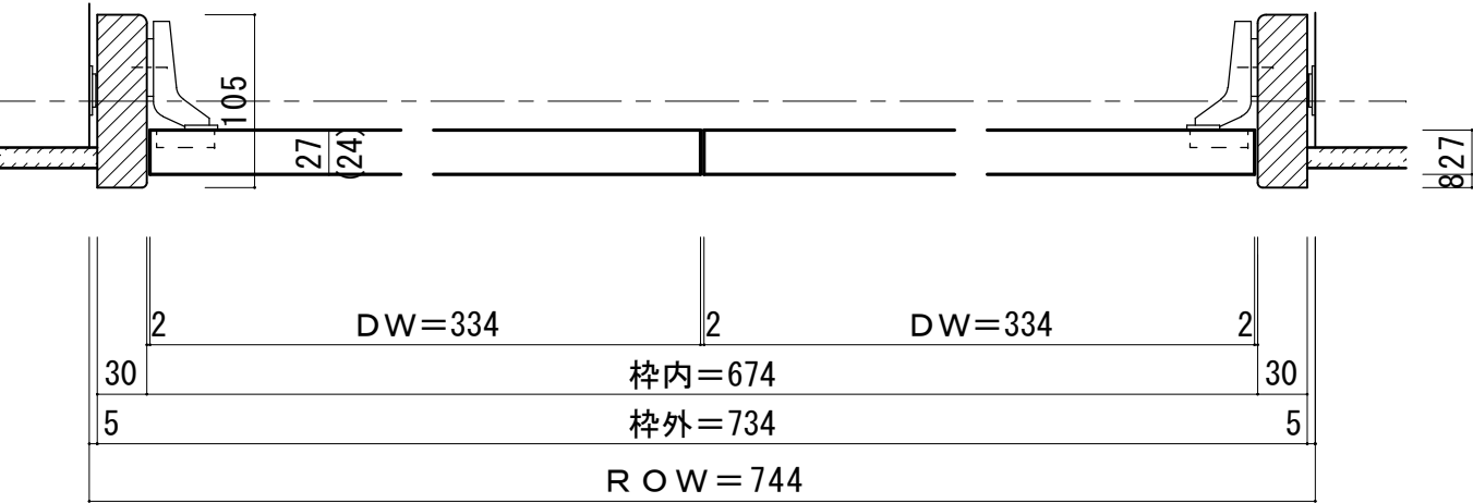
■横断面図 H=8尺、7尺、6尺
