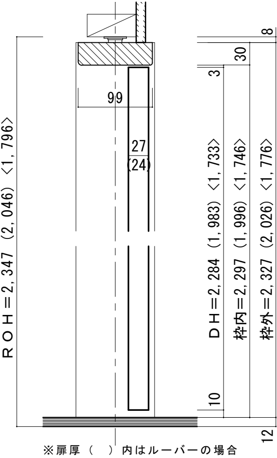
■縦断面図 H=8尺 (7尺) <6尺>
