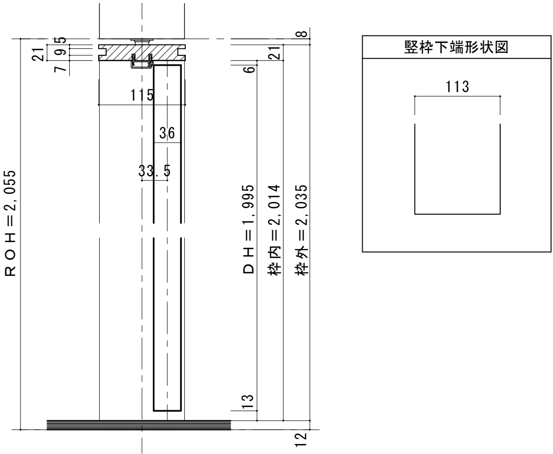
■ 縦断面図
