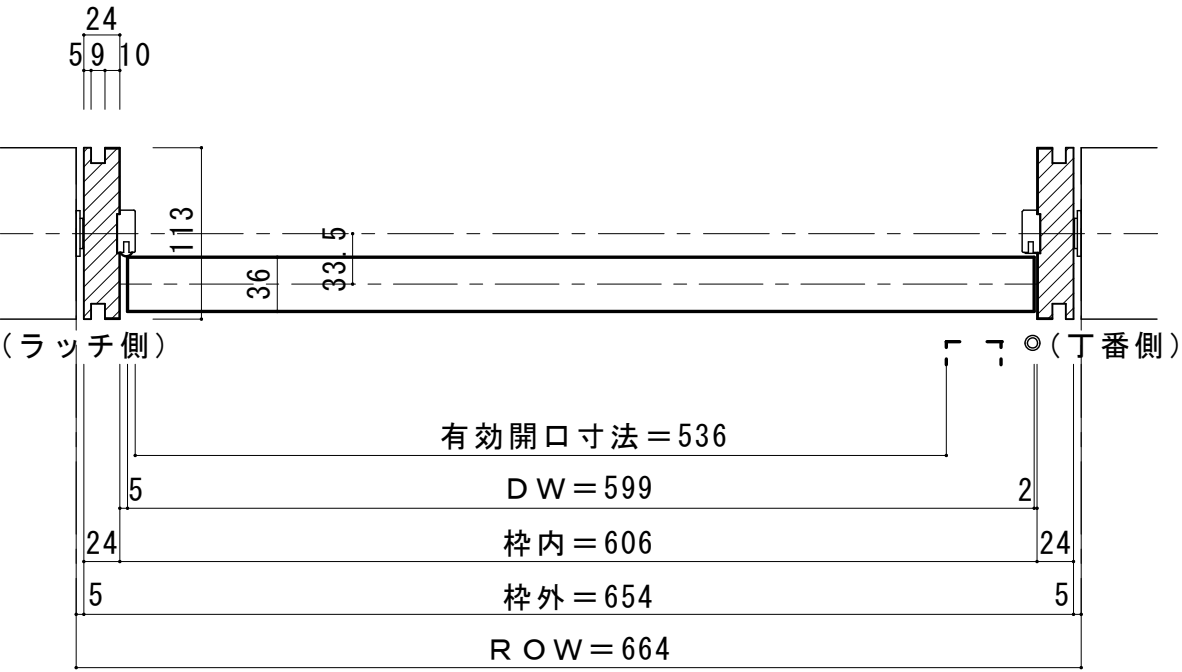
■横断面図 ※図示：右吊り元
