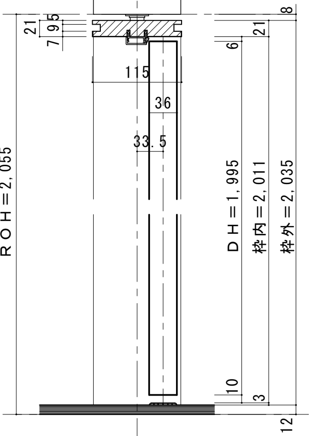
■縦断面図 [床直付けレール]
