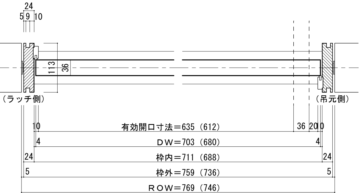
■横断面図
