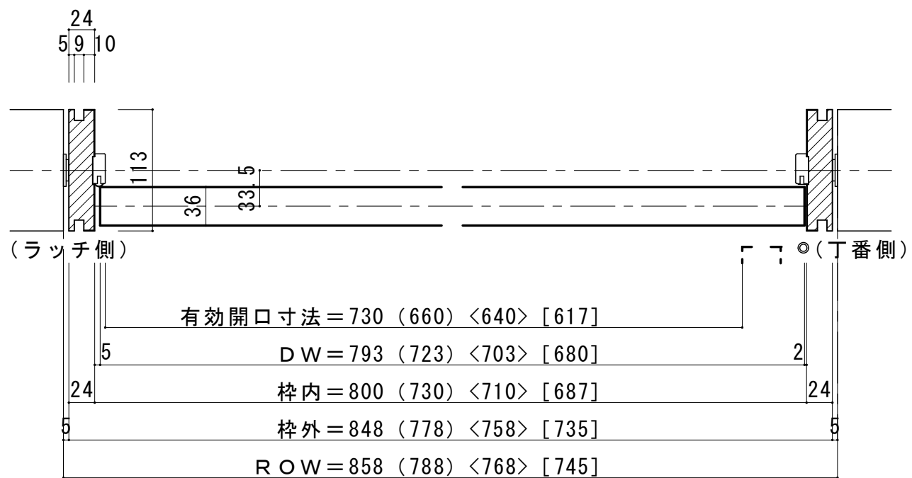
■ 横断面図 ※図示：右吊り元
