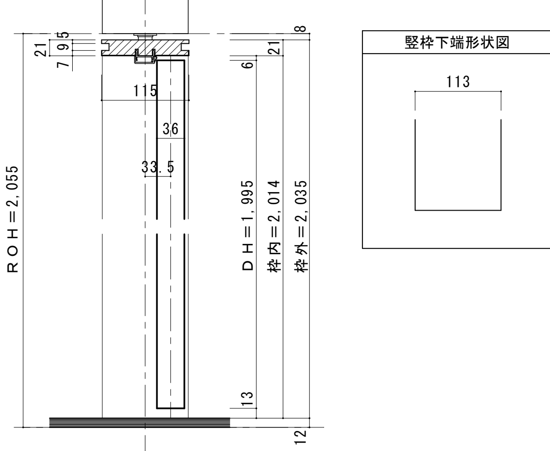
■ 縦断面図
