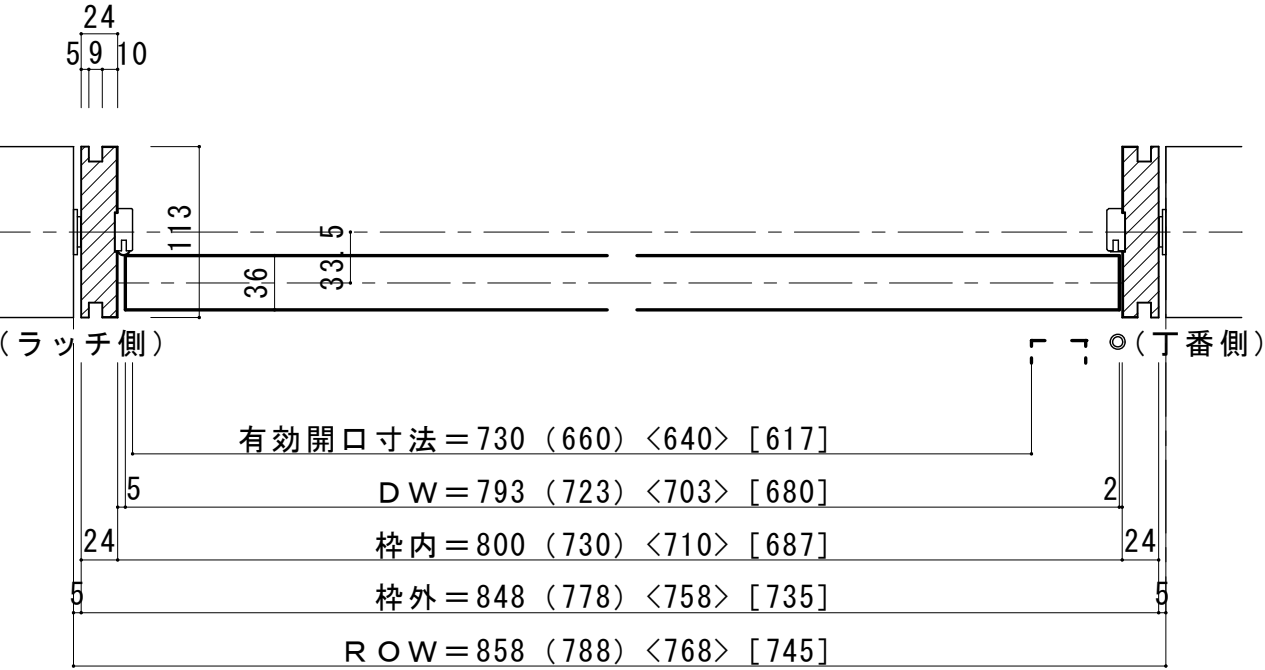
■横断面図
