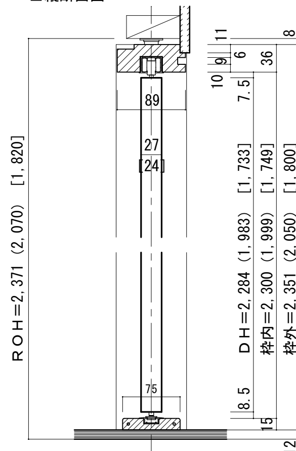
■縦断面図
