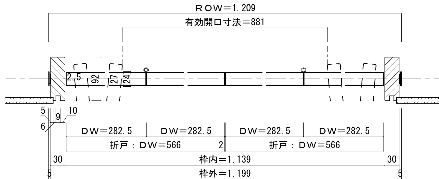
■横断面図
