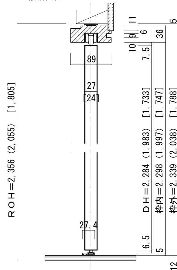
■縦断面図
