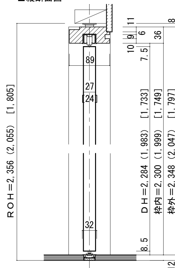
■縦断面図
