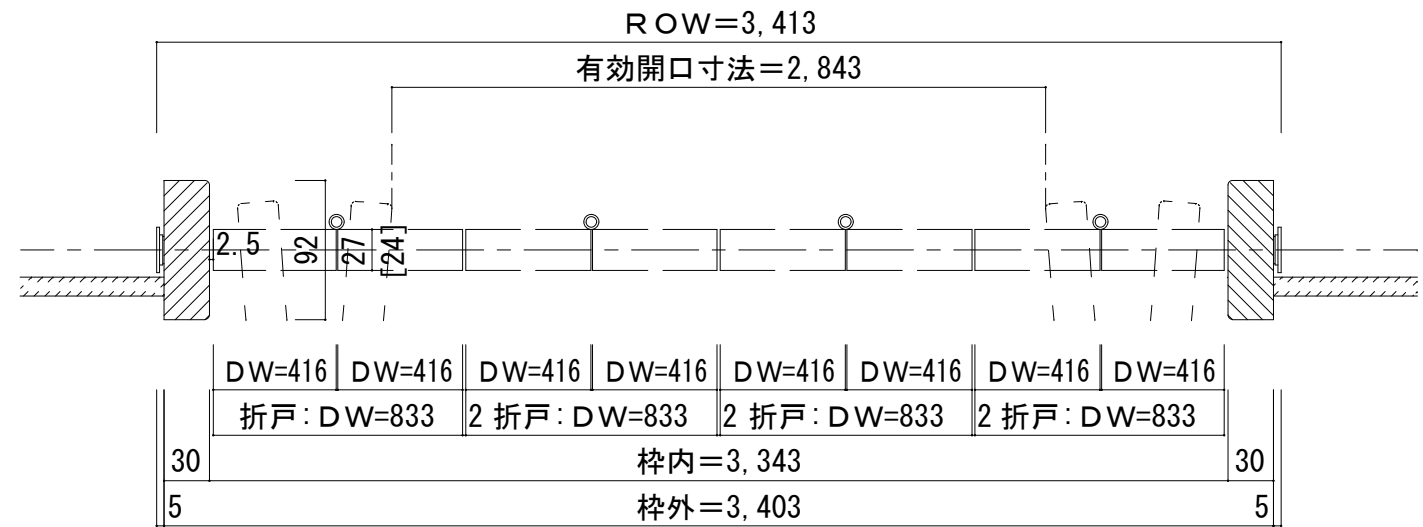
■横断面図
