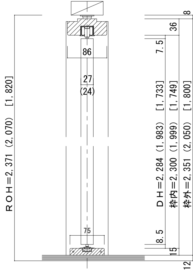
■縦断面図
