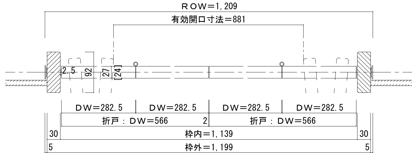
■横断面図
