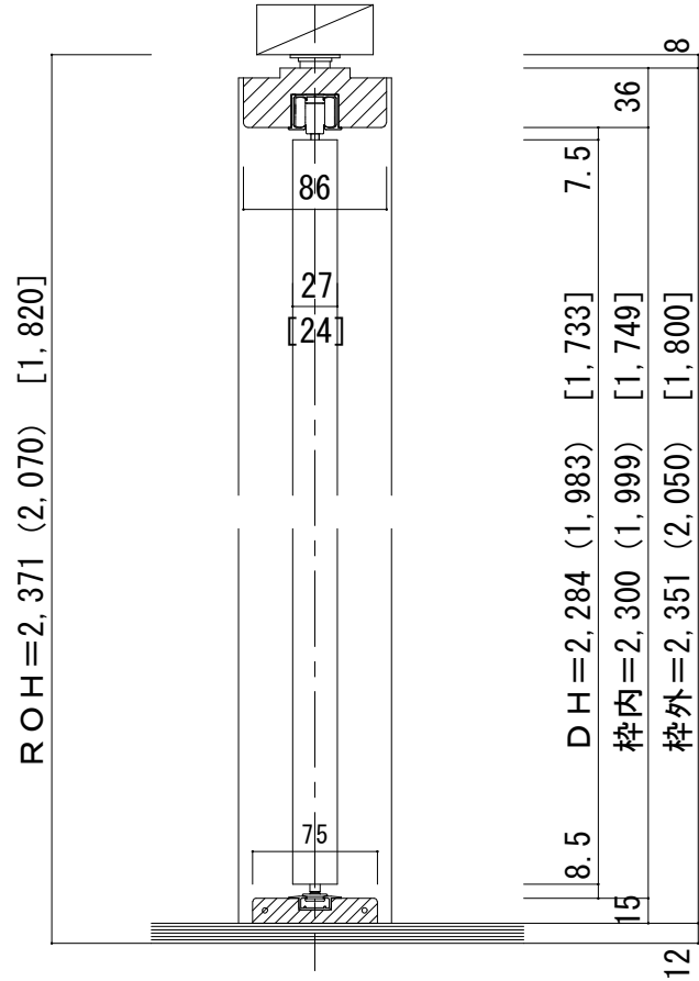
■縦断面図
