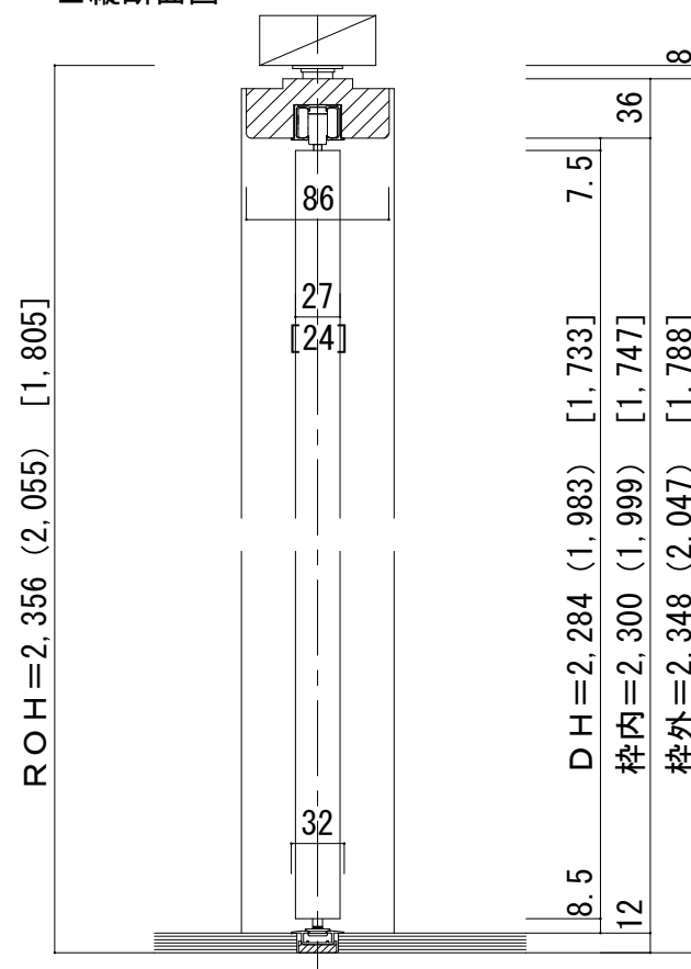
■縦断面図
