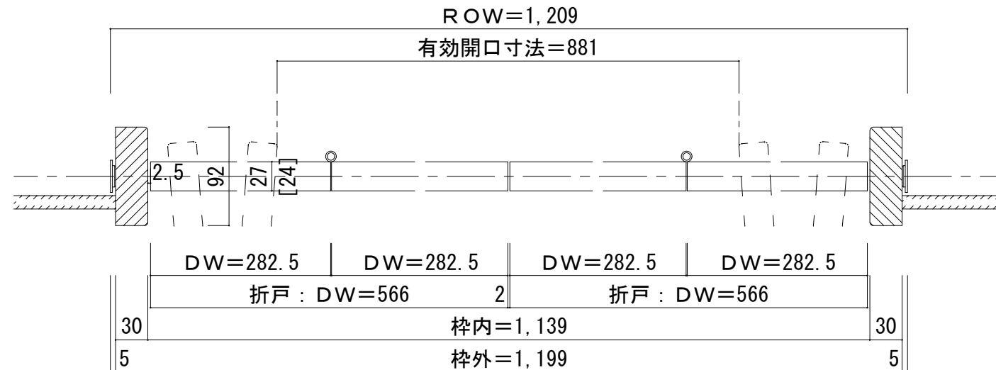
■横断面図
