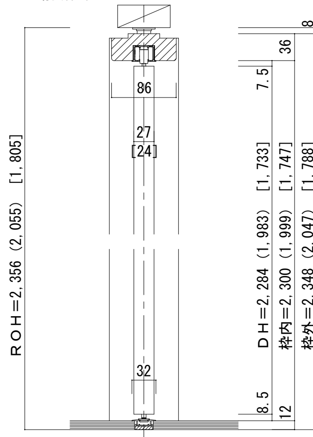
■縦断面図
