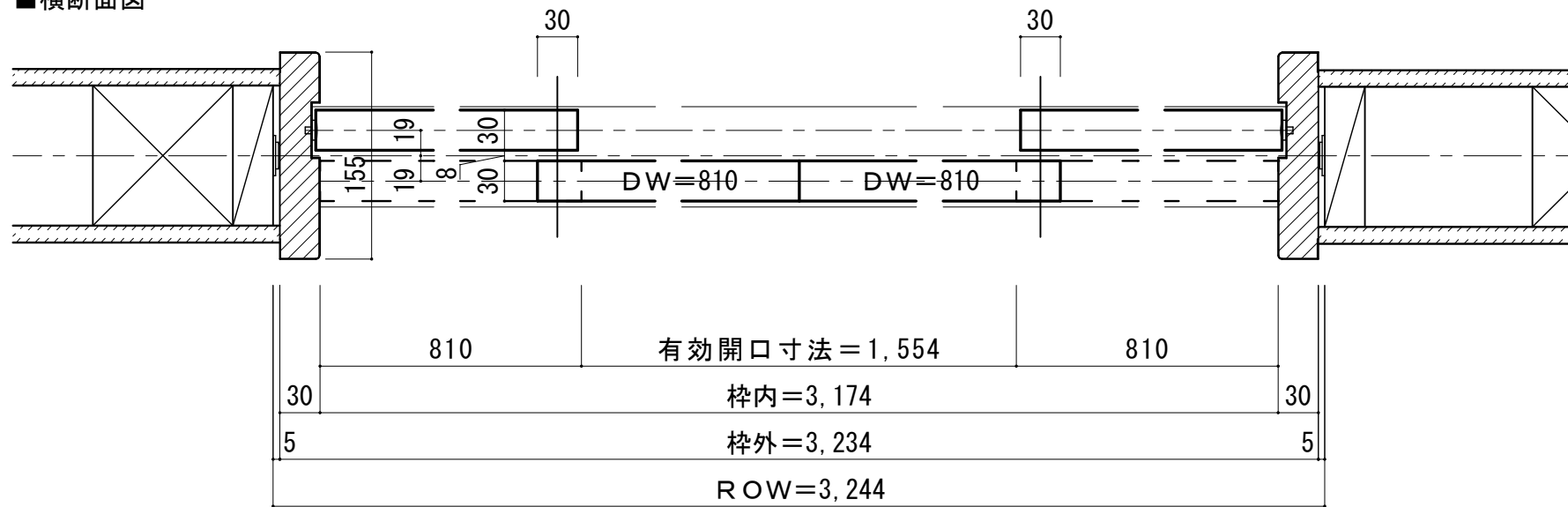
■横断面図
