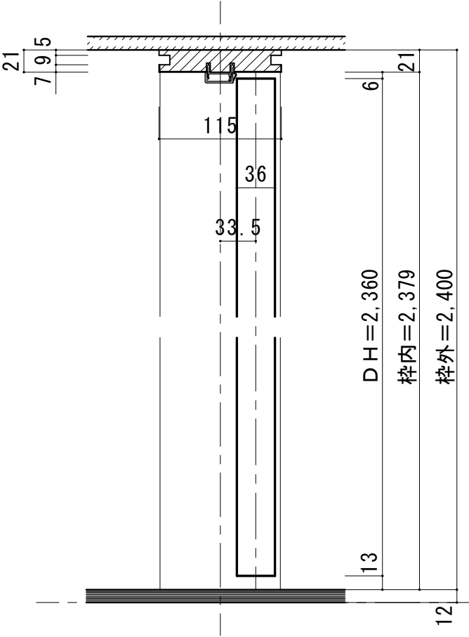
■ 縦断面図
