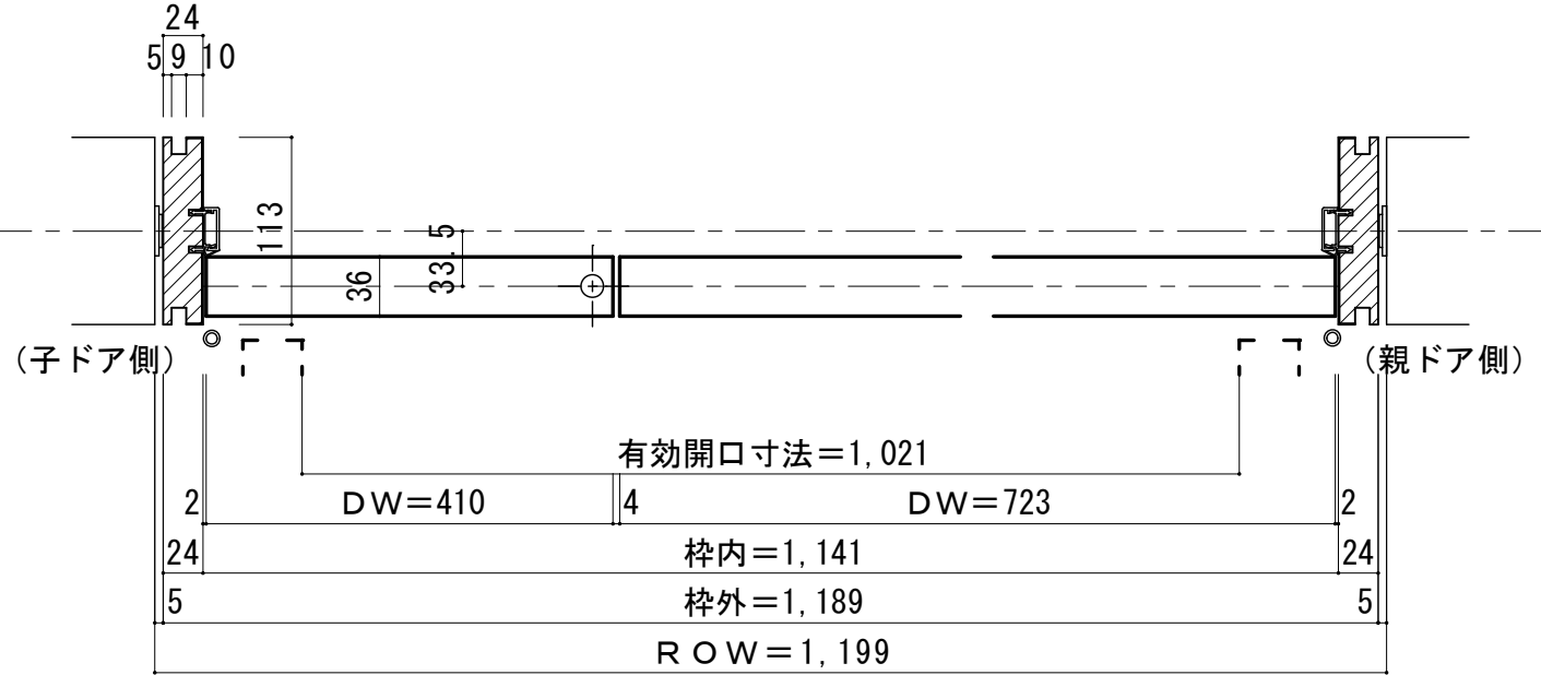
■ 横断面図 ※図示：右吊り元
