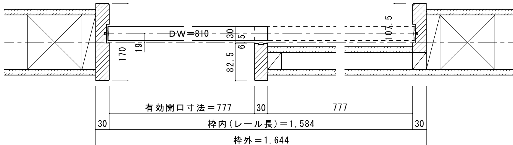
■横断面図 ※図示：左引き手
