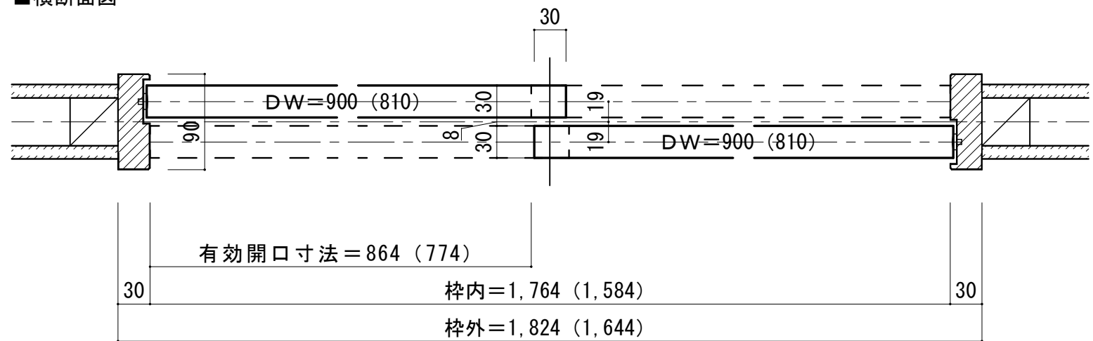
■横断面図
