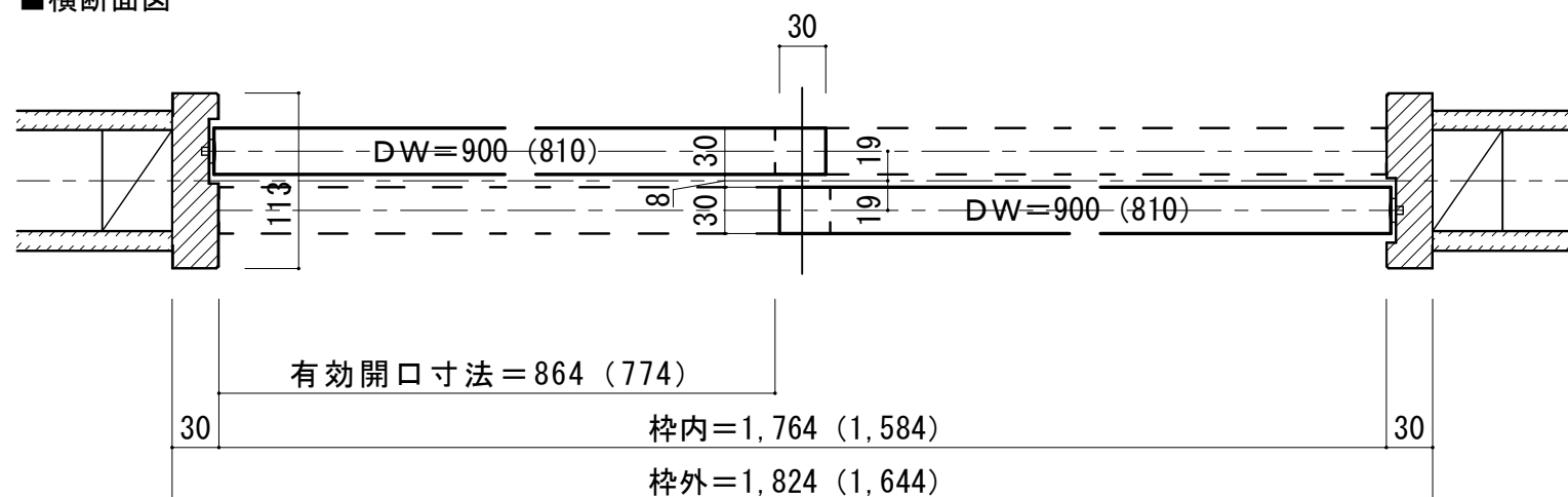
■横断面図
