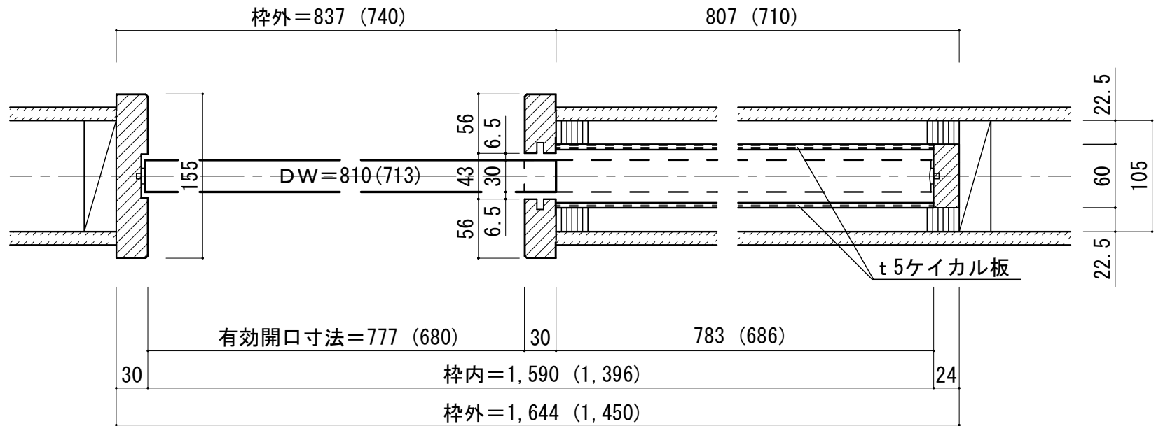
■横断面図
