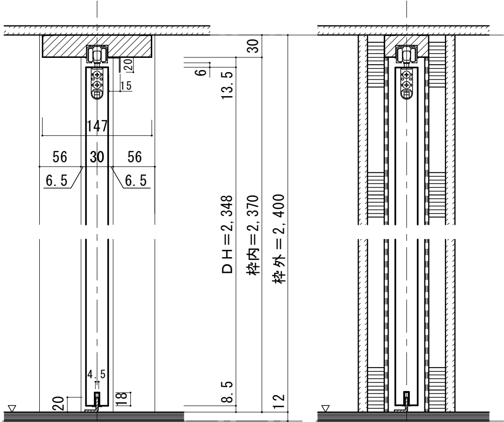
■縦断面図
