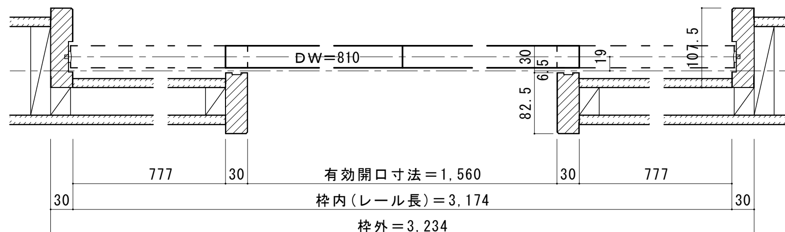
■横断面図
