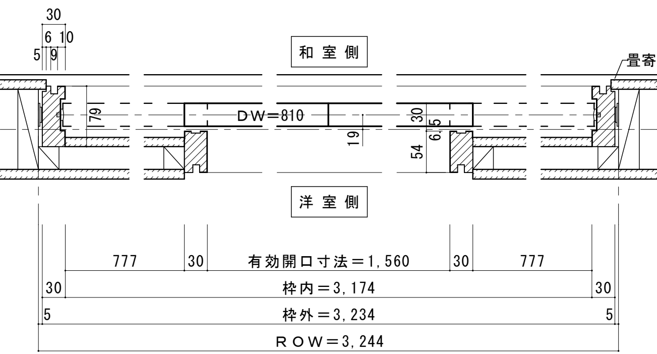
■横断面図
