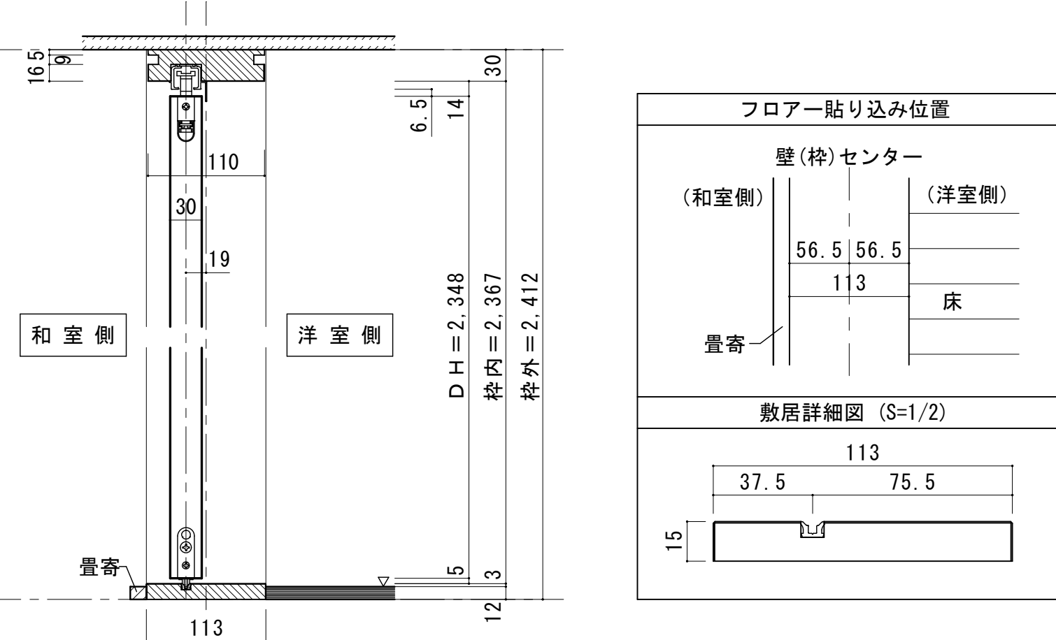
■縦断面図
