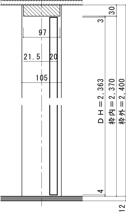
■縦断面図
