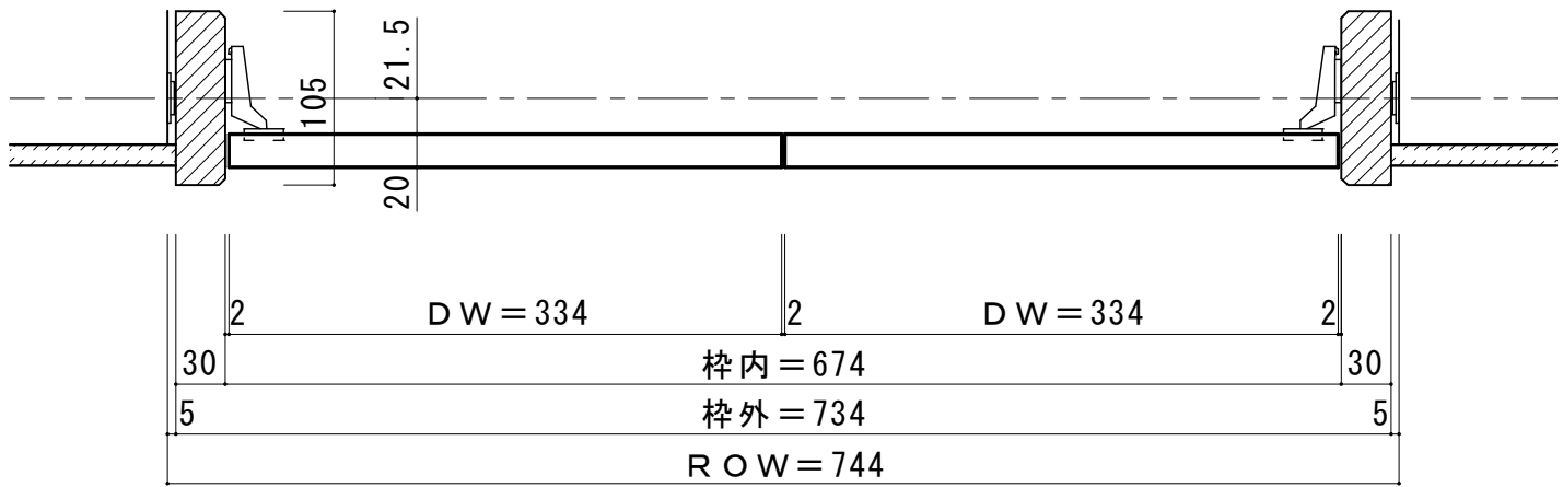
■横断面図
