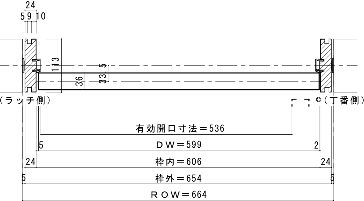
■横断面図 ※図示：右吊り元
