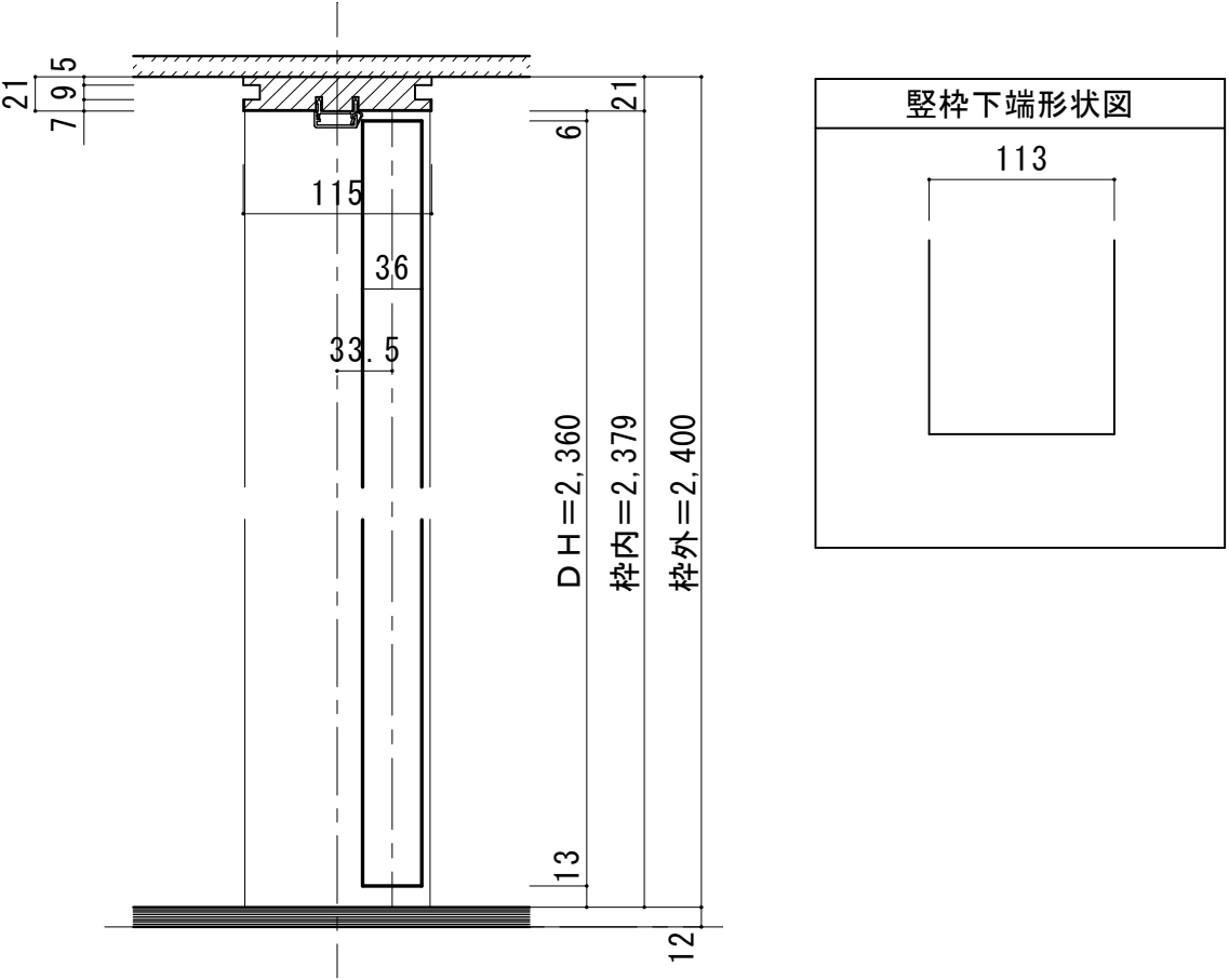
■縦断面図
