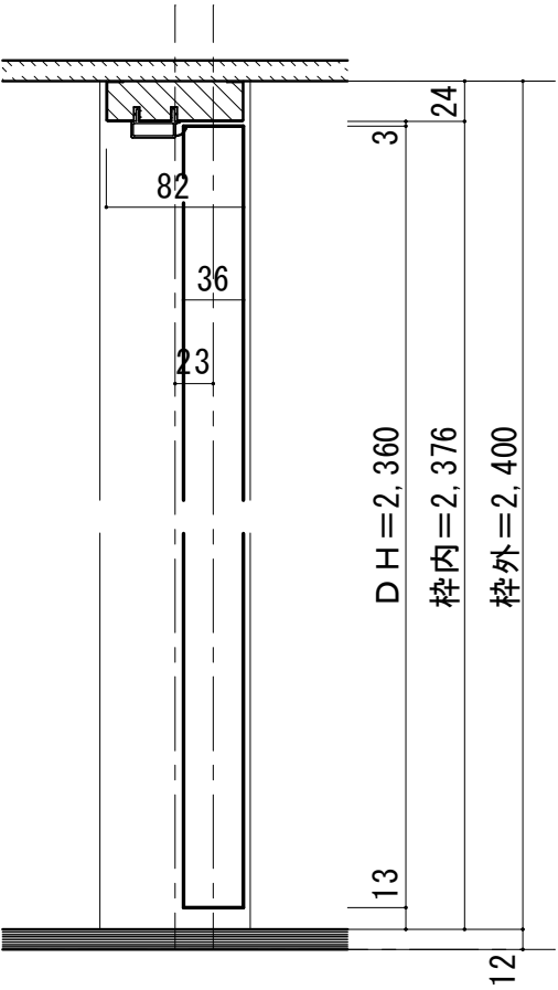
■ 縦断面図
