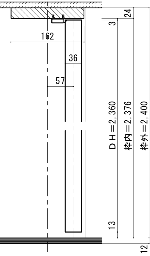
■縦断面図
