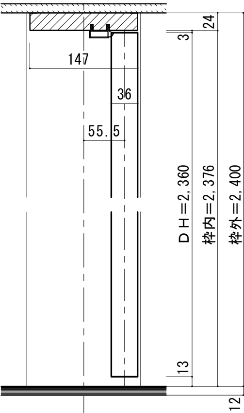
■ 縦断面図
