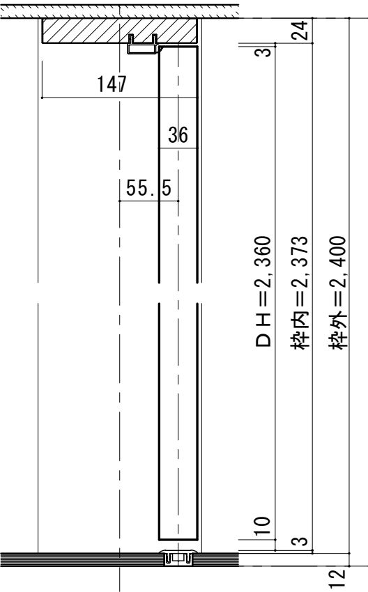
■ 縦断面図 [両ツハタイプ]
