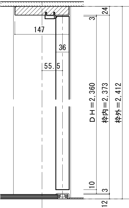
■ 縦断面図 [片ツハタイプ]
