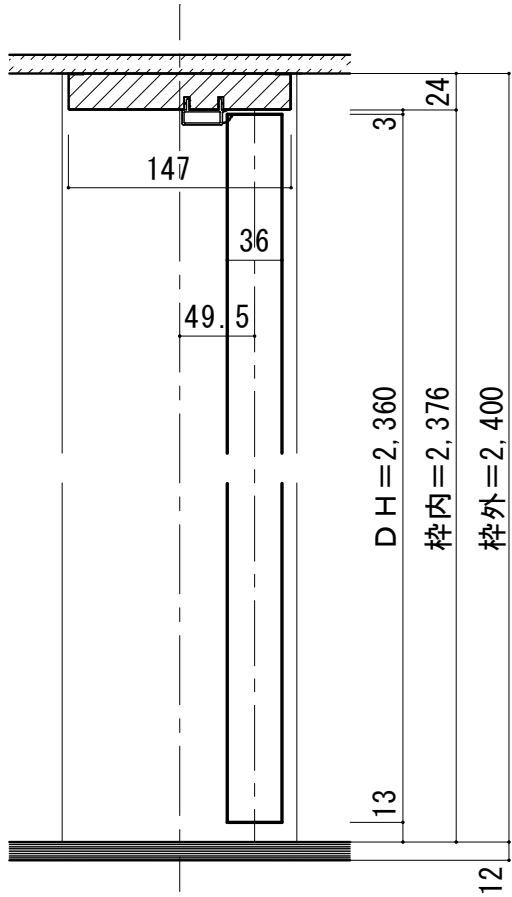
■ 縦断面図
