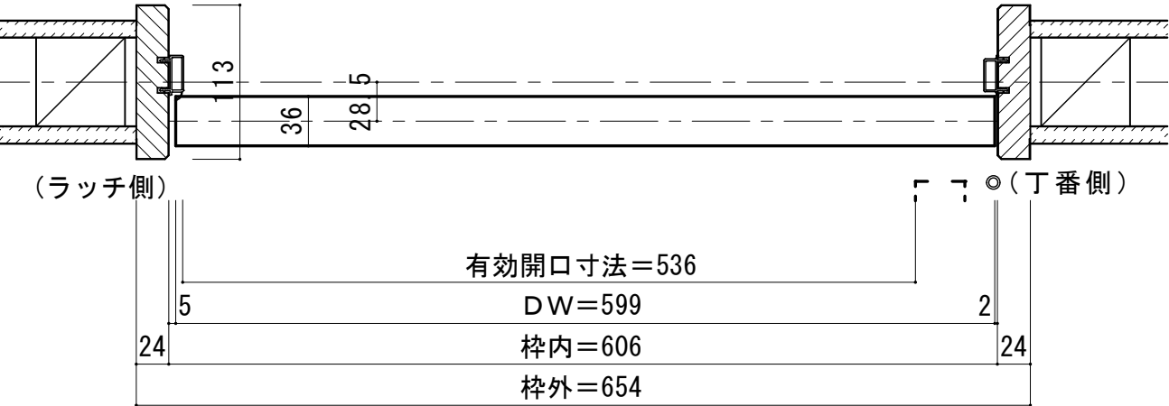
■ 横断面図 ※図示：右吊り元
