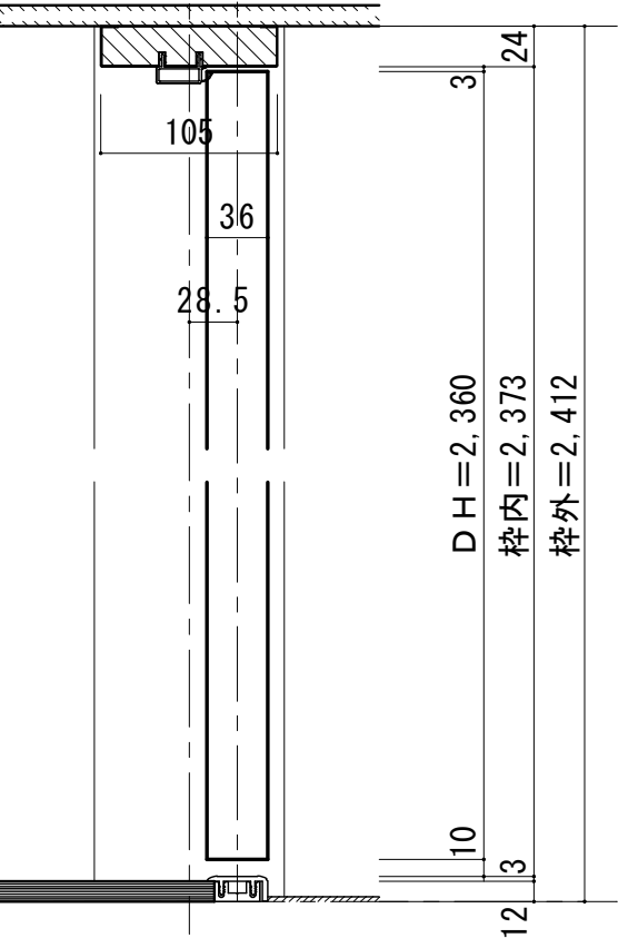
■ 縦断面図 [片ツハタイプ]
