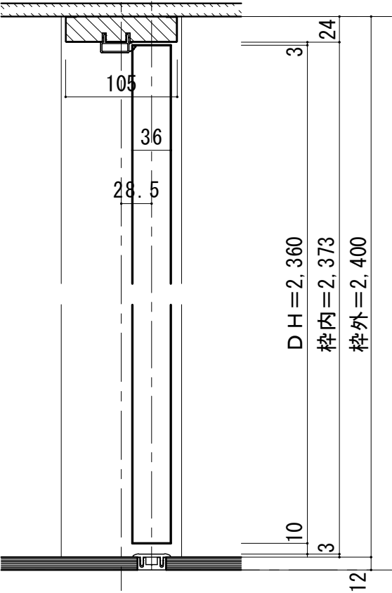
■ 縦断面図 [両ツハタイプ]
