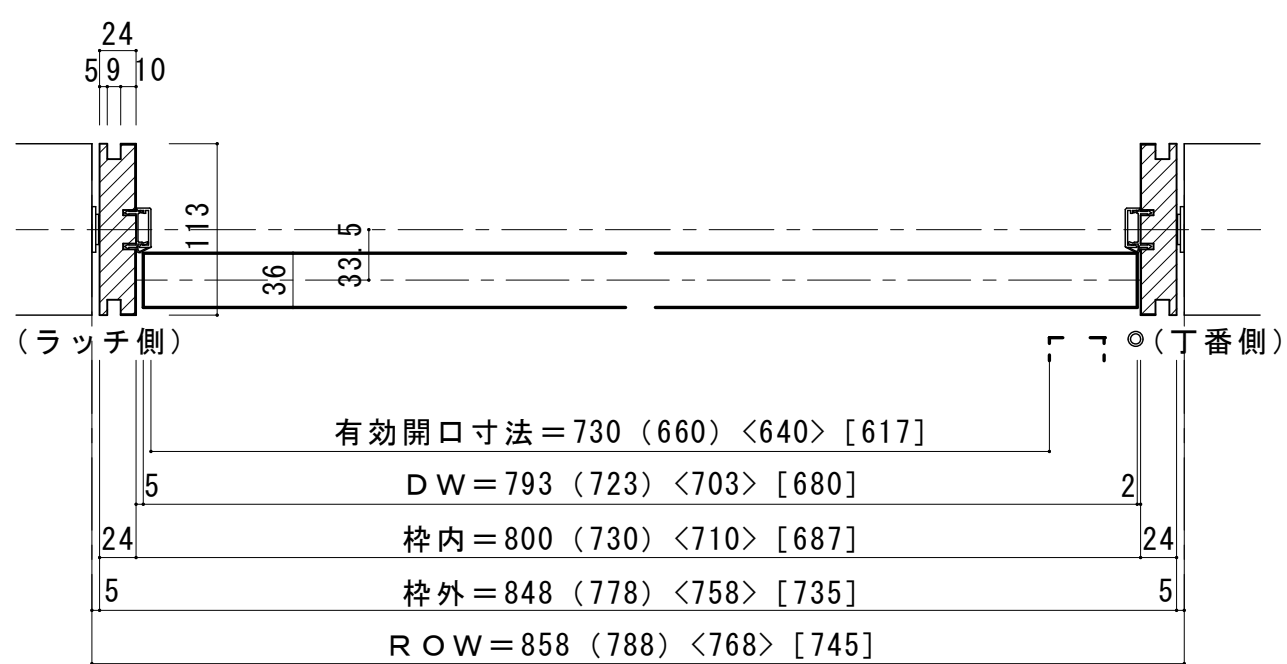
■横断面図 ※図示：右吊り元
