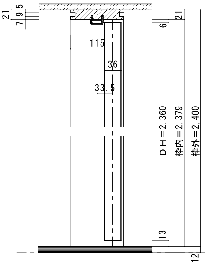
■縦断面図
