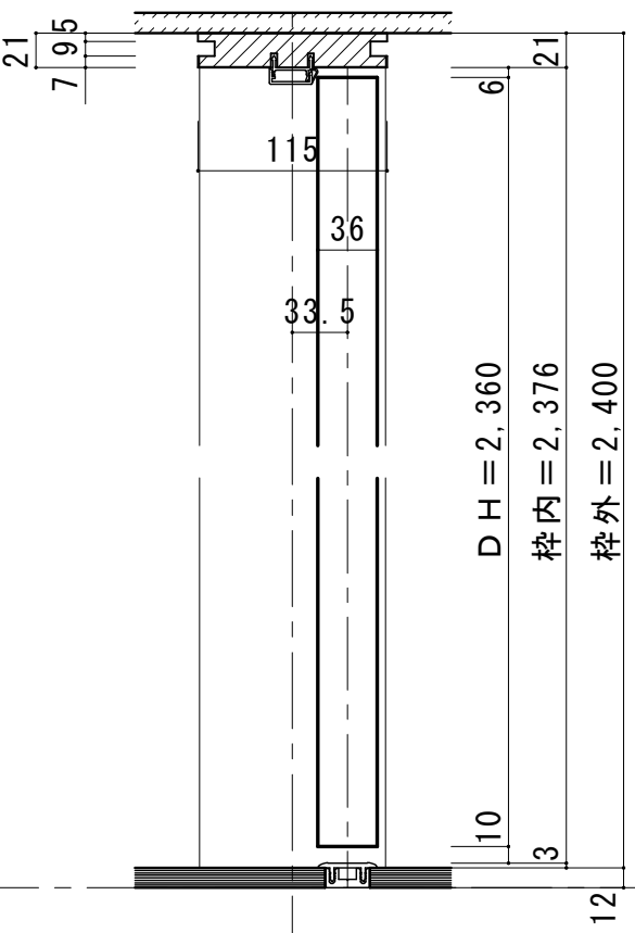
■縦断面図 [両ツパタイプ]
