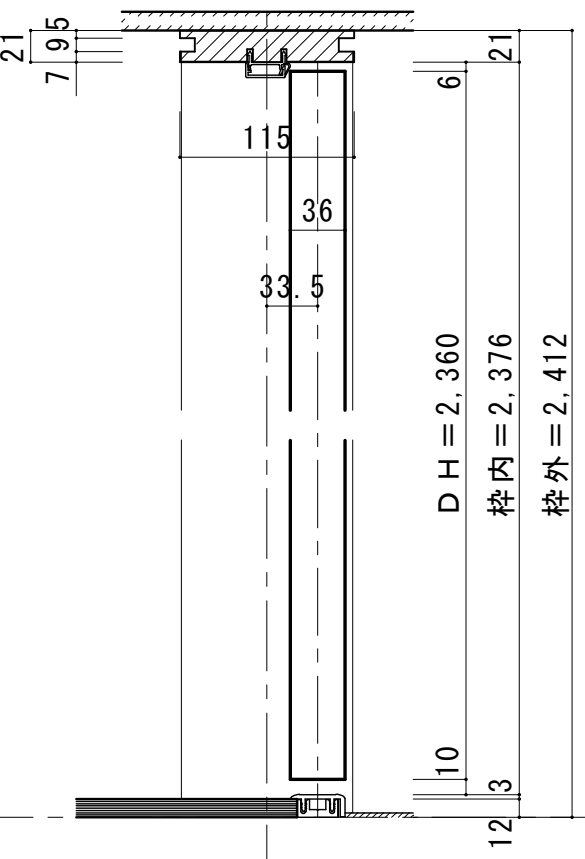
■縦断面図 [片ツパタイプ]
