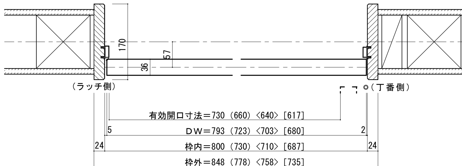
■ 横断面図 ※図示：右吊り元
