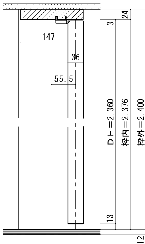
■縦断面図
