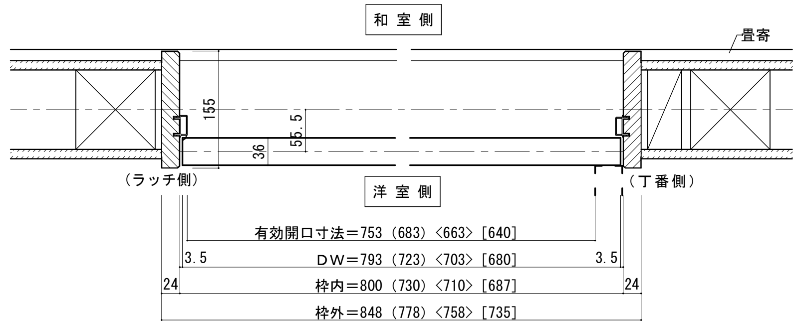
■ 横断面図 ※図示：右吊り元
