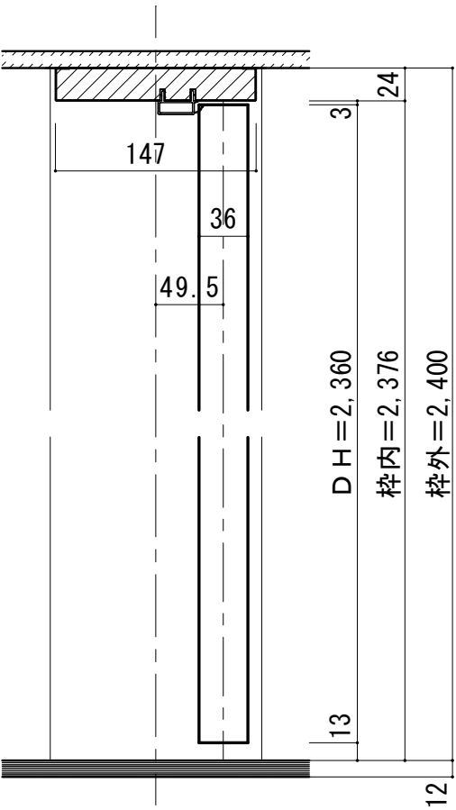
■ 縦断面図
