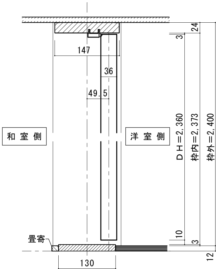
■縦断面図
