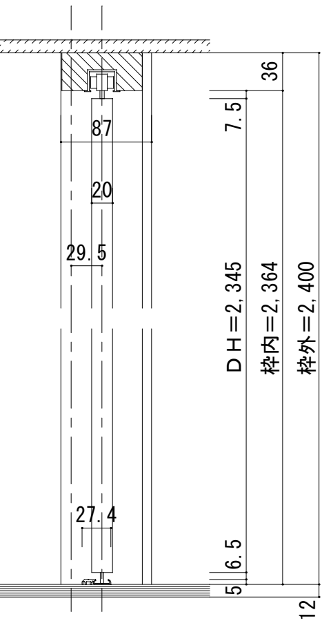
■縦断面図
