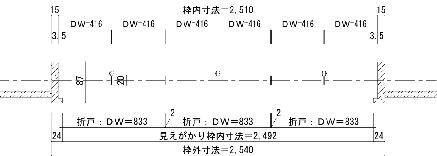
■横断面図
