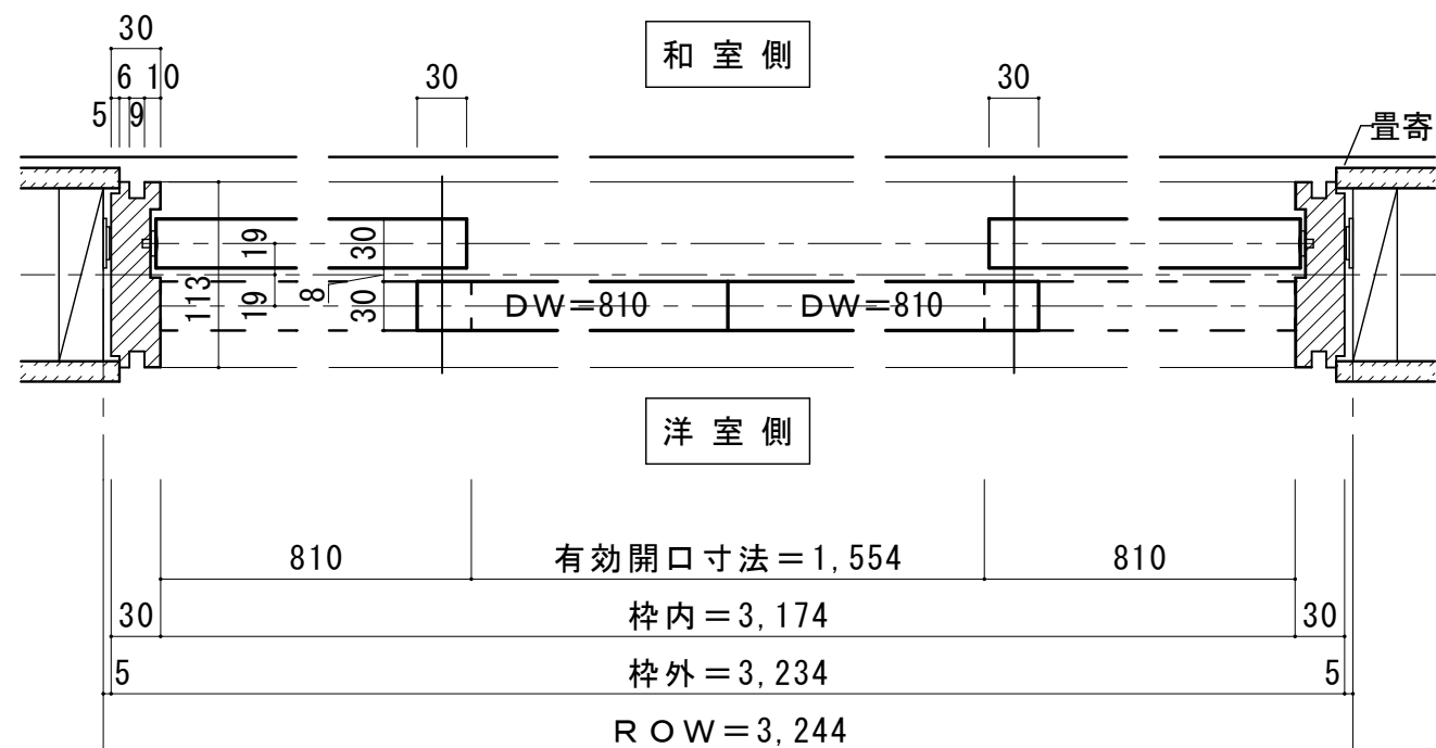
■横断面図
