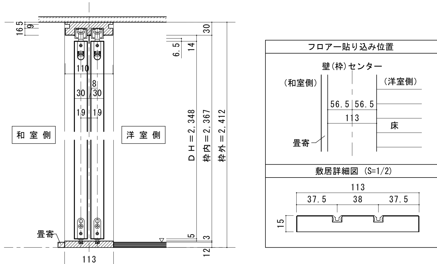
■縦断面図
