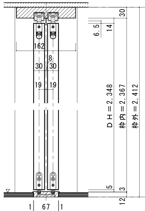
■縦断面図[敷居Q型]
