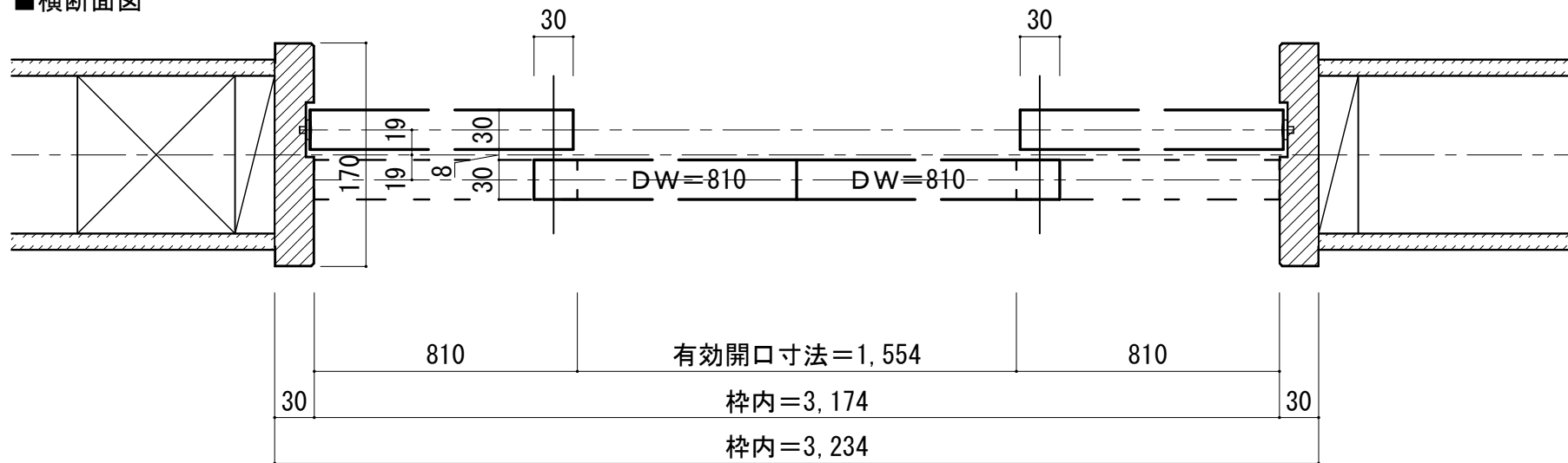
■横断面図
