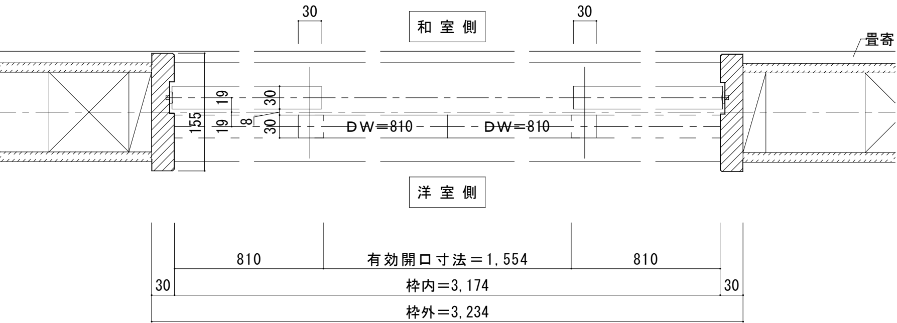
■横断面図
