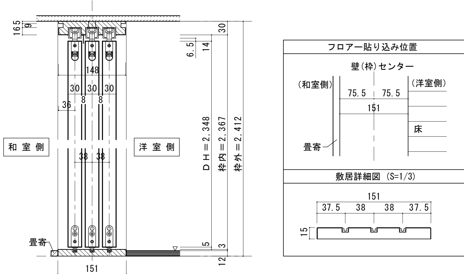
■縦断面図
