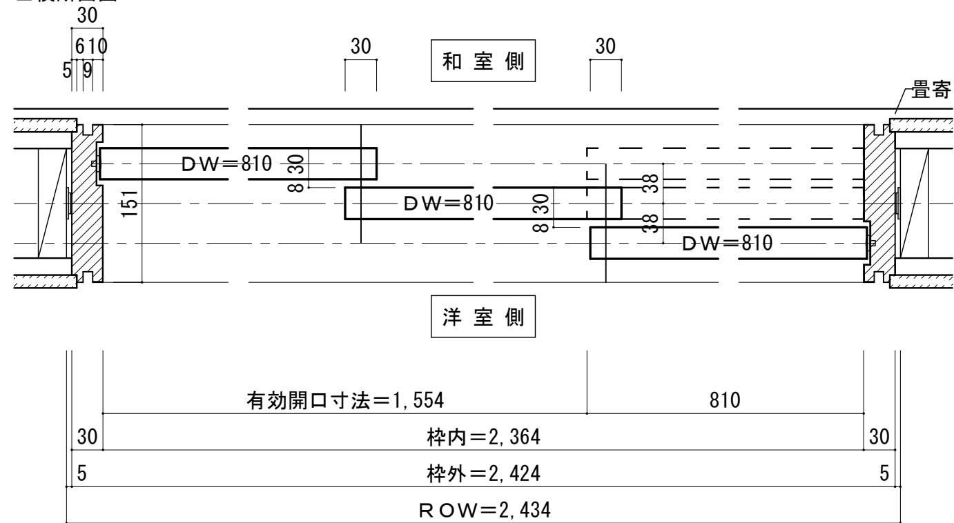
■横断面図
