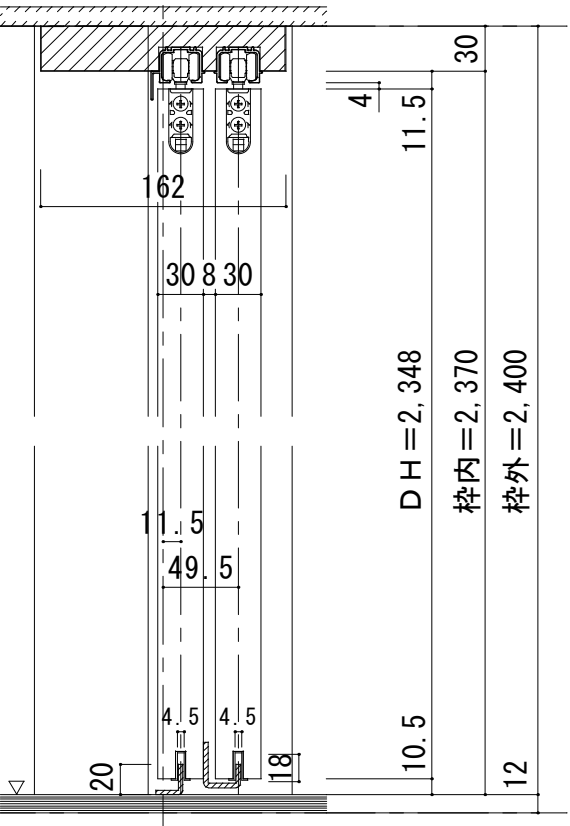
■縦断面図
