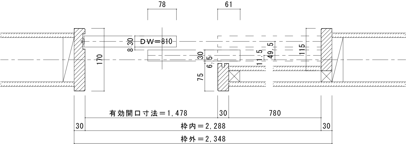
■横断面図 ※図示：左引き手
