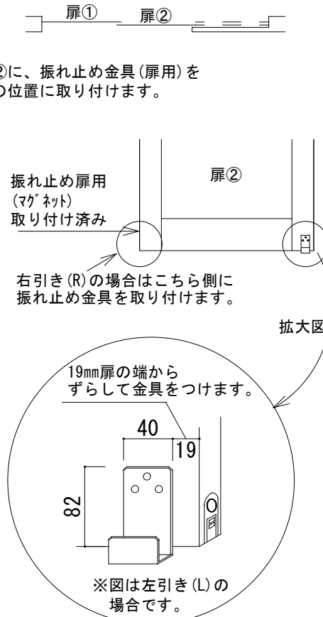
振れ止め金具(扉付け用)取り付け
