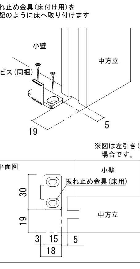
振れ止め金具(床付け用)取り付け
