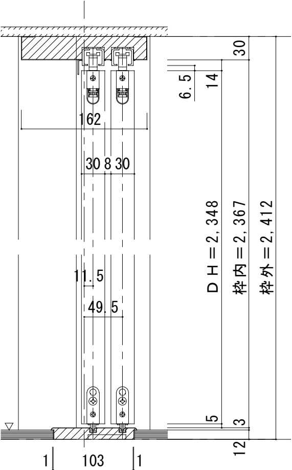
■縦断面図[敷居Q型]
