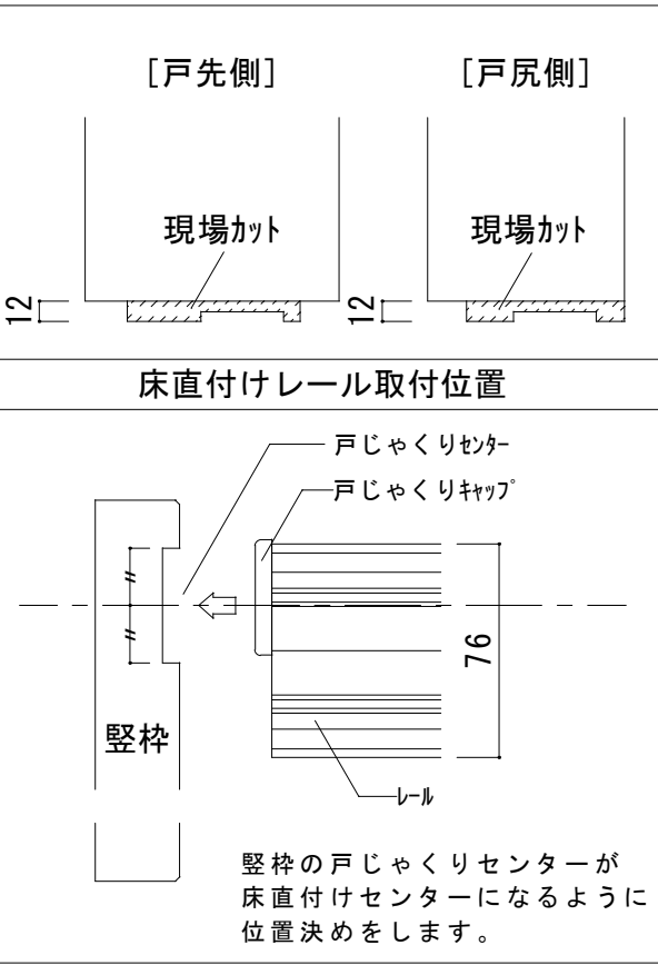
■縦枠下端加工図
