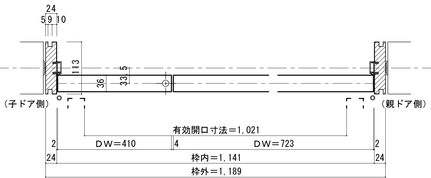
■横断面図 ※図示：右吊り元
