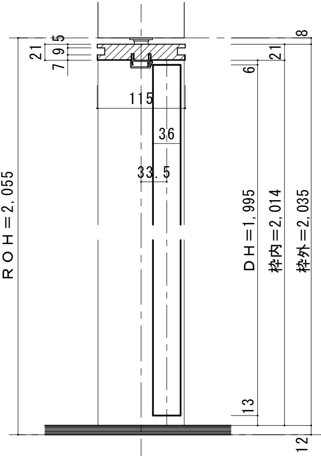
■縦断面図
