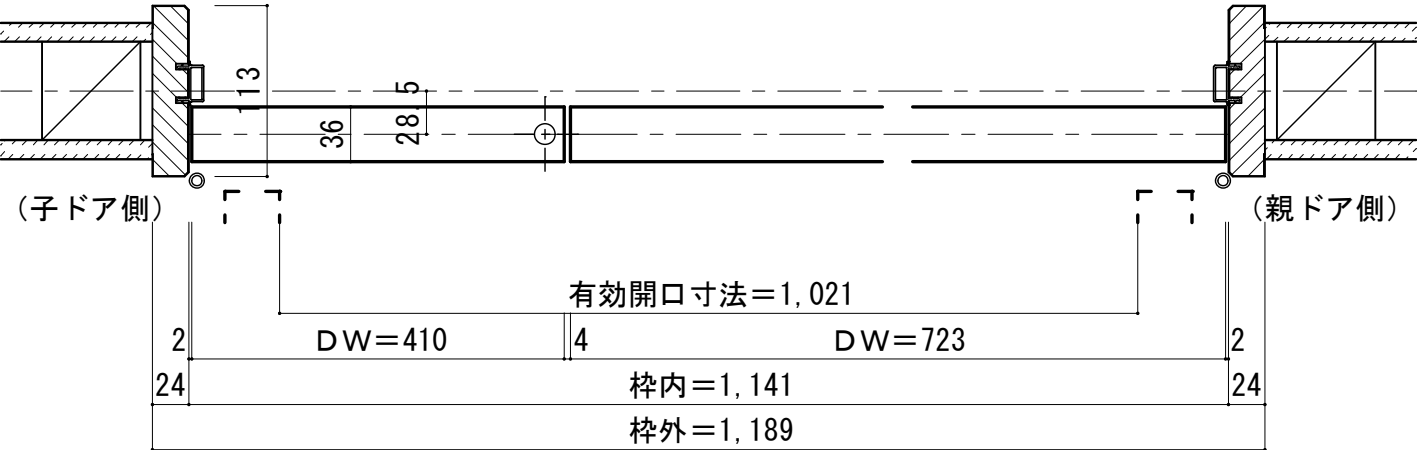
■ 横断面図 ※図示：右吊り元
