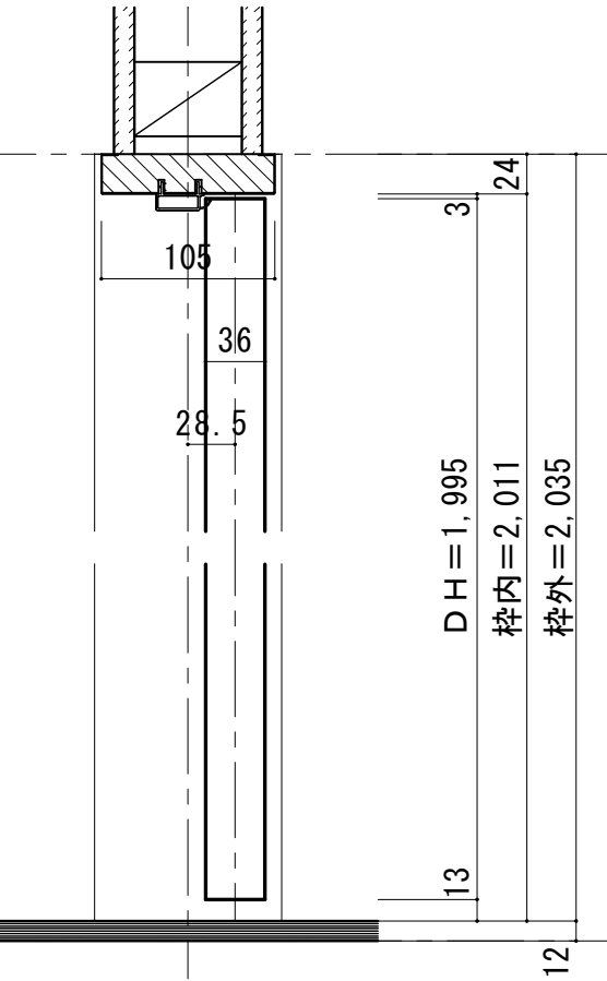
■ 縦断面図
