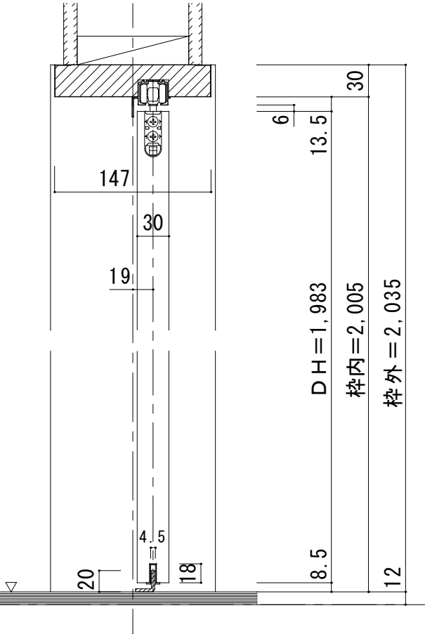
■縦断面図
