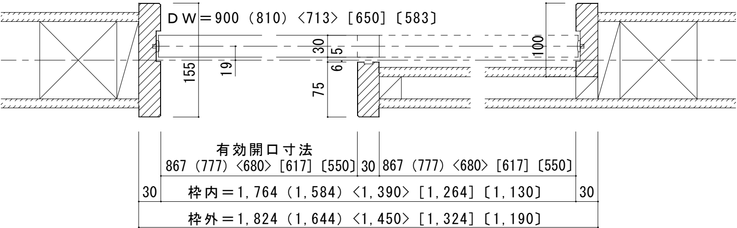
■横断面図 ※図示：左引き手
