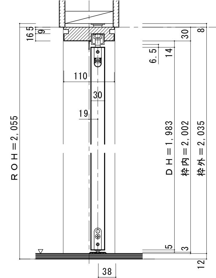
■縦断面図[床直付けレール]
