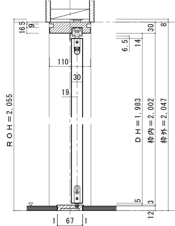
■縦断面図[敷居Q型]
