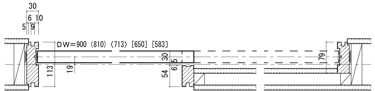
■横断面図 ※図示：左引き手
