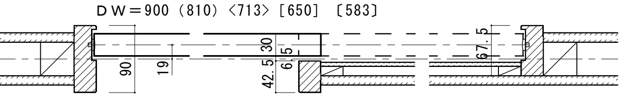
■横断面図 ※図示：左引き手
